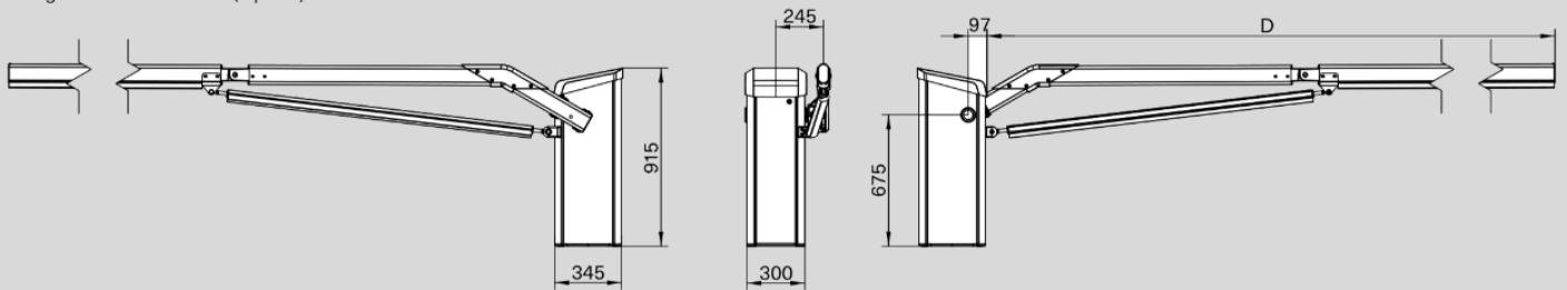
Parking Pro mit Knickbaum (Option)
