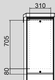
Terminal-MXL Detailansicht Frontplatte 310
