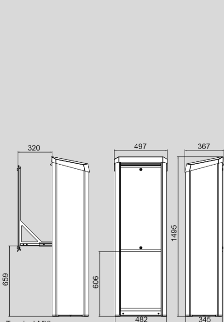
Terminal-MXL Ansicht von der Seite mit ausgefahrener Frontplatte, von vorne und von der gegenüberliegenden Seite
