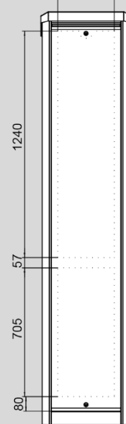
Terminal-MXXL Detailansicht Frontplatte
